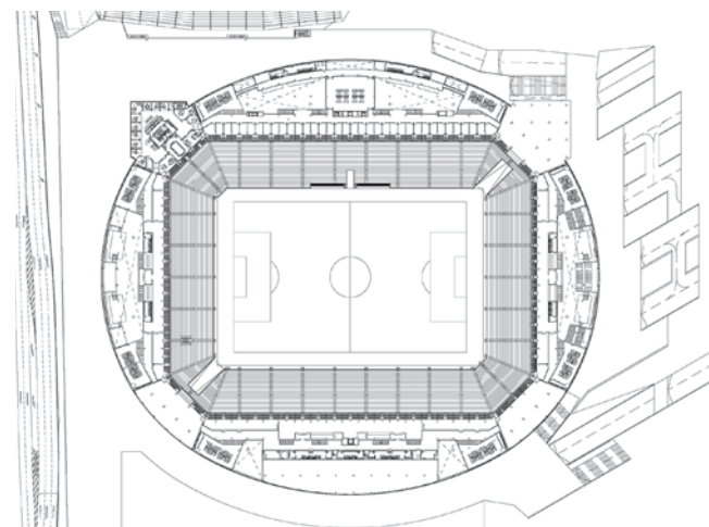
Pianta del livello VIP
